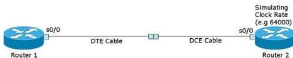
crossover DTE/DCE cable
